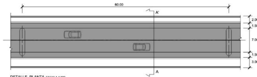
DETALLE PLANTA ESCALA 1/400
