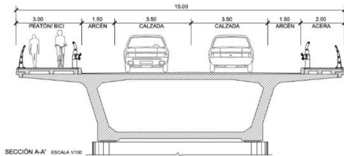
SECCIÓN A-A' ESCALA 1/100
