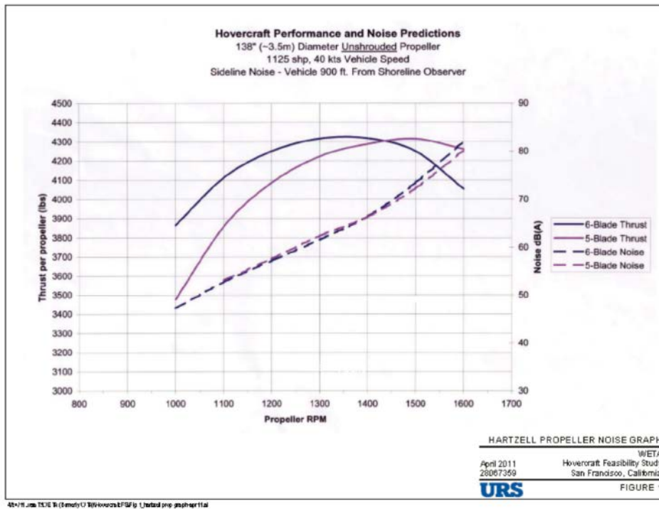
-Gráfico 1- Niveles de Ruido propulsor tipo "Hartzell" 117
