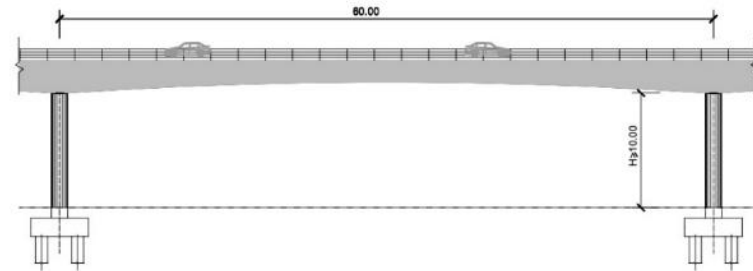
DETALLE ALZADO ESCALA 1/400
