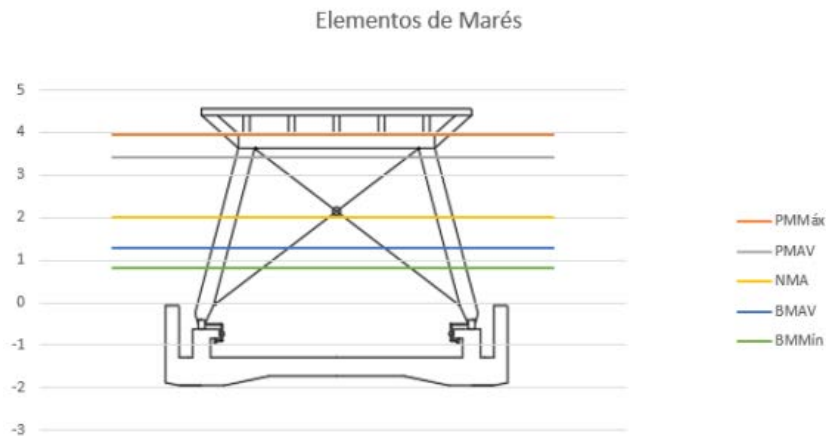
Figura 4.2 - Esquema explicativo das cotas de projeto
